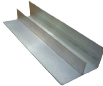
Polymer F Profile/ Aluminium F Profile Length : 4 Meter Thickness : 20 mm, 30 mm Order Code : 20 FPR, 30 FPR 20 AFPR, 30 AFPR
